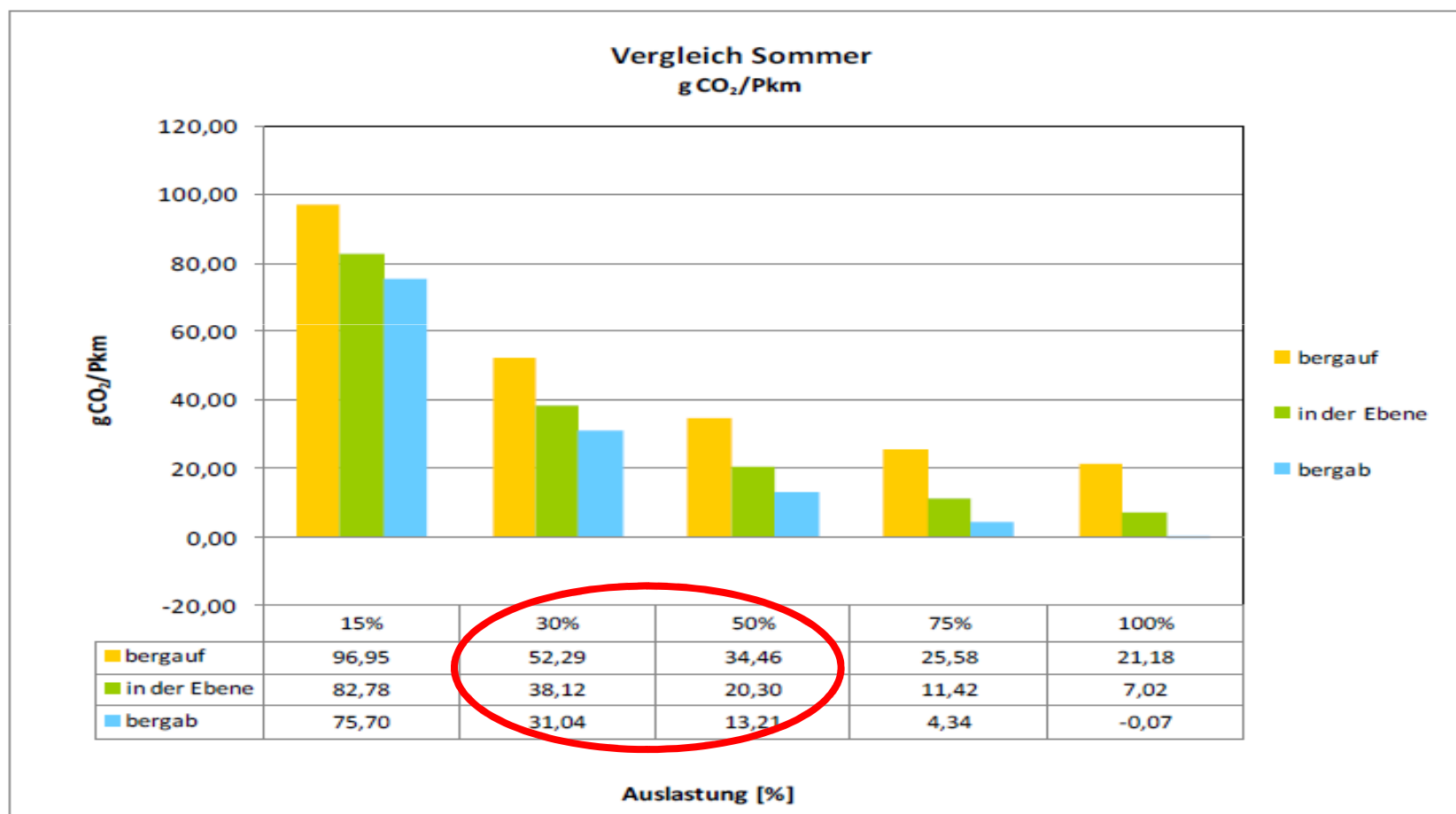
Abbildung 3 Vergleich Sommer-Seilbahnen
